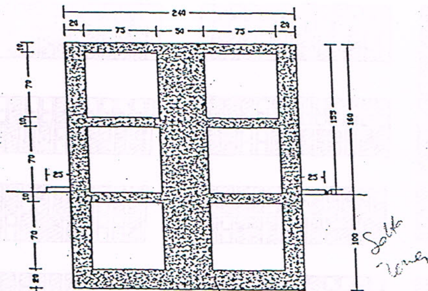
SEZIONE A-A
