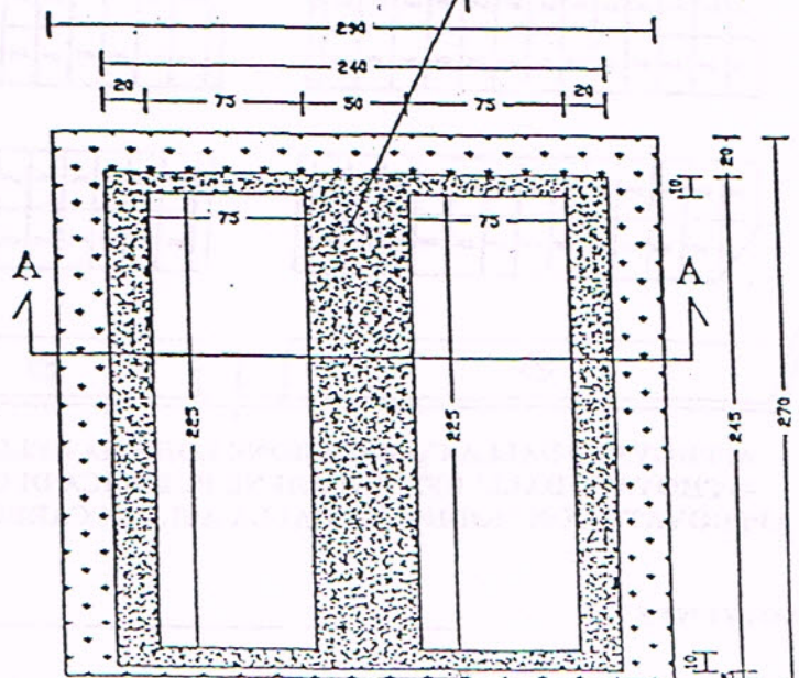
PIANTA
